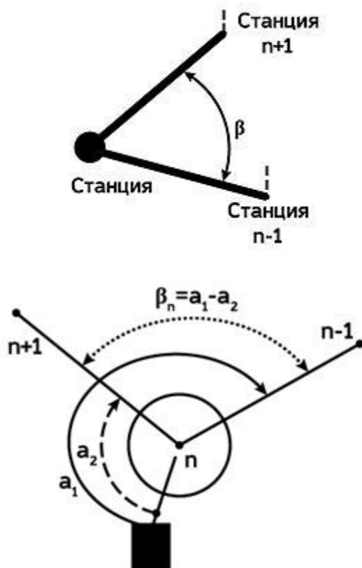
Рисунок 3. Измерение горизонтального угла на станции.
