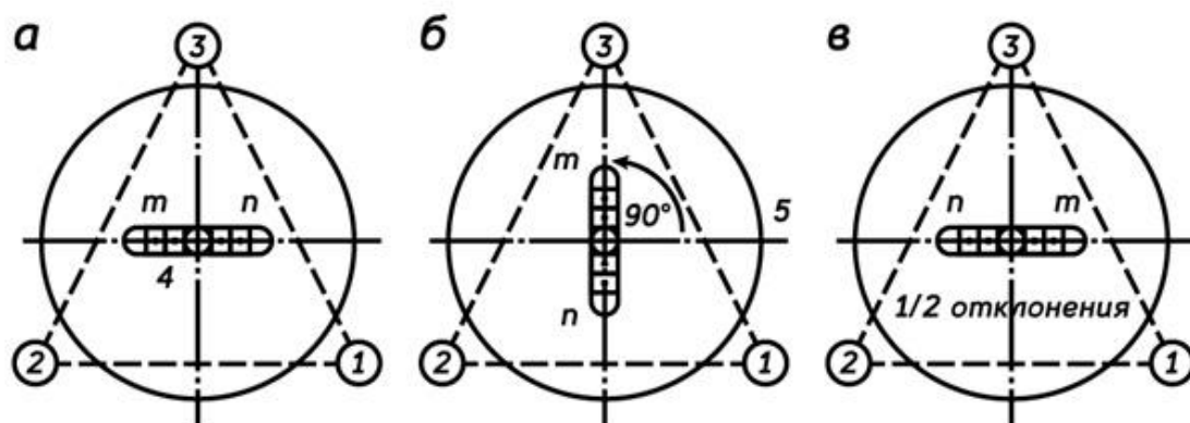
Рисунок 1. Горизонтирование теодолита
