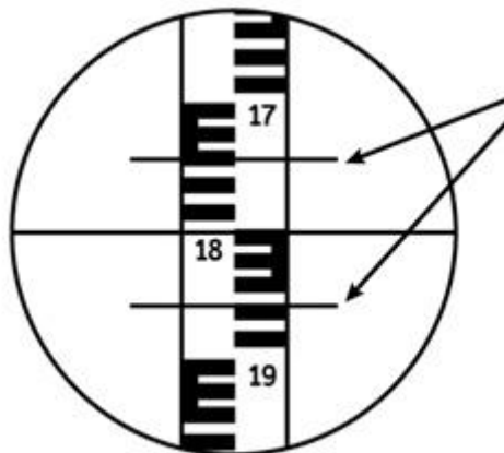
Рисунок 4. Определение расстояния по дальномеру
