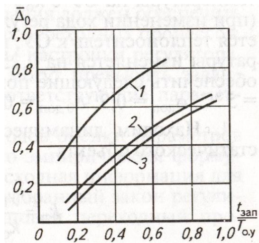
Рис. 2.68. Графики изменения относительной статической ошибки \bar{\Delta}_0 от величины t_{\text{зап}}/T_{o.y} :
