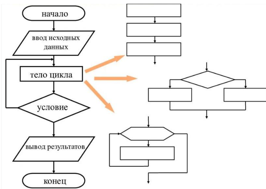
Примеры составления блок-схем циклической структуры
