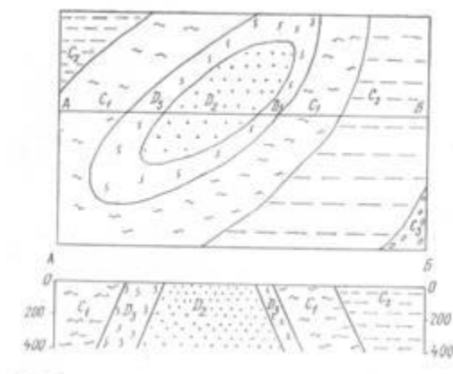
Геологический разрез
