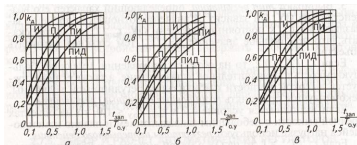
Рис. 2.67. Графики изменения динамических коэффициентов регулирования k_d для статических объектов от величины t_{\text{зап}}/T_{0.у} :
