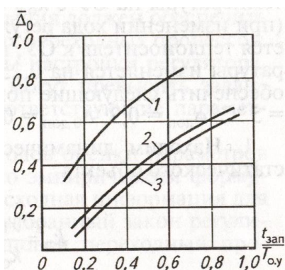
Рис. 2.68. Графики изменения относительной статической ошибки \bar{\Delta}_0 от величины t_{\text{зап}}/T_{0.у} :
