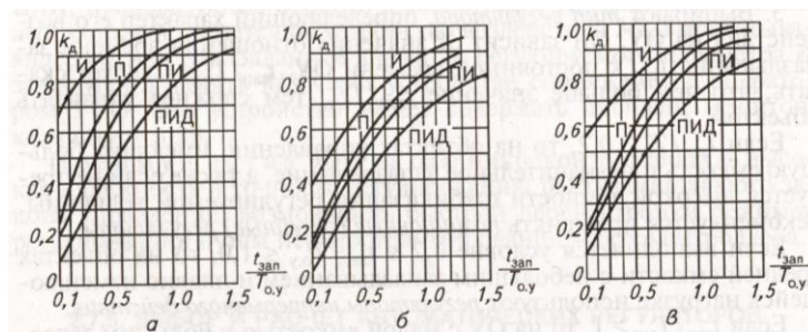
Рис. 2.67. Графики изменения динамических коэффициентов регулирования k_d для статических объектов от величины t_{\text{зап}}/T_{0,y} : а — для аperiodических переходных процессов; б — для процессов с 20%-ным перерегулированием; в — для процессов с минимумом интегральной оценки J_2
